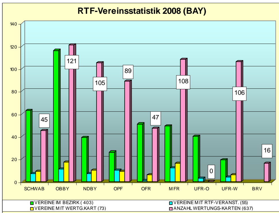
Abb.2 RTF-Verein-Statistik 2008
